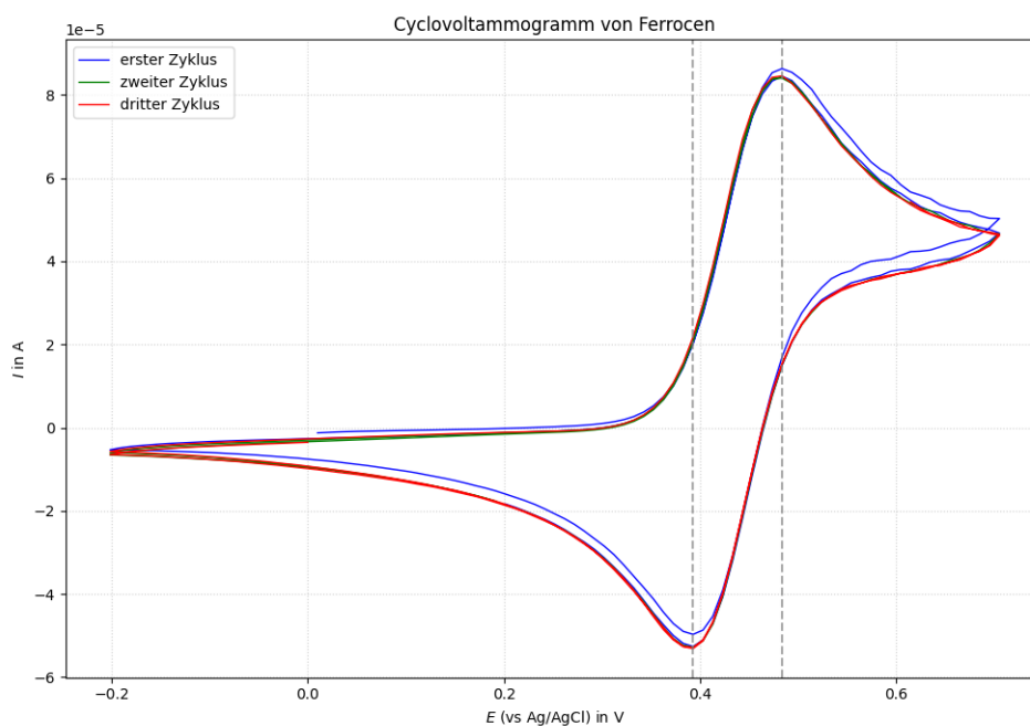
Abb. 4: Die Abbildung zeigt das CV von einem Ferrocen/Ferrocenium Zusatz mit einer \text{Ag}/\text{AgCl} -Elektrode als Gegenelektrode. Die gestrichelten Linien sind dabei E_{\text{max}} , E_{\text{min}} .
